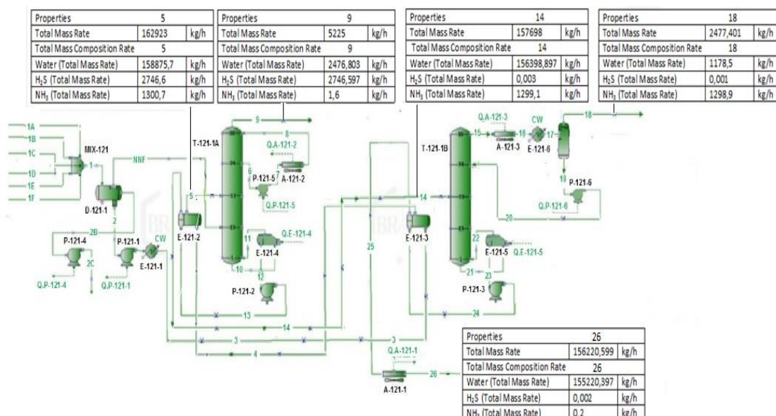
Figura 1. Modelo de simulación de las torres recuperadoras.
